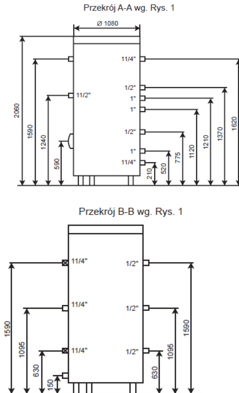
Rys. 2 Wymiary podgrzewacza
