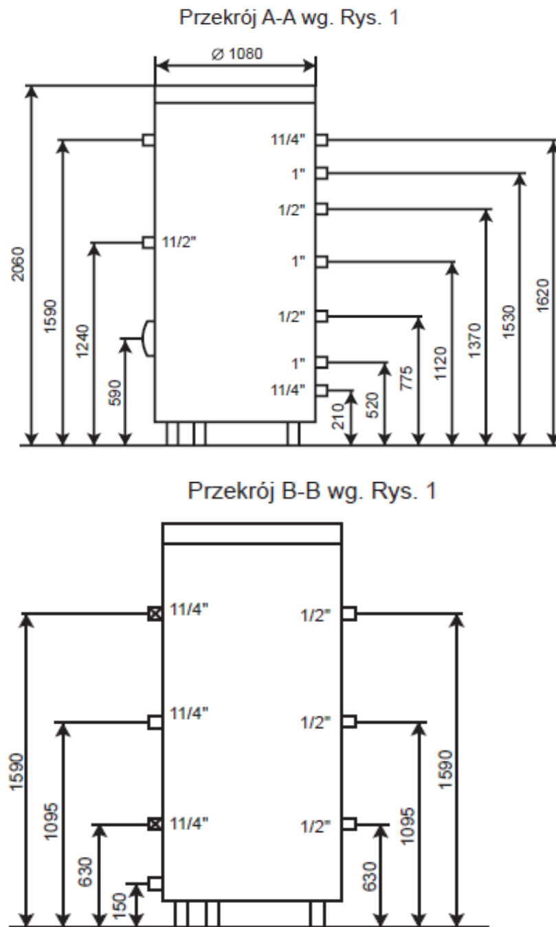
Rys. 2 Wymiary podgrzewacza
