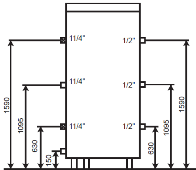
Rys. 2 Wymiary podgrzewacza
