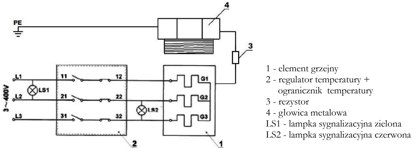
Rys. 4 Schemat elektryczny podgrzewacza z grzałką elektryczną 3- fazową
