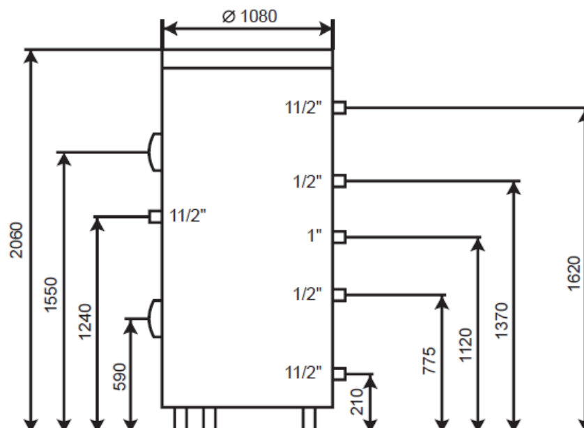
Przekrój A-A wg. Rys. 1
