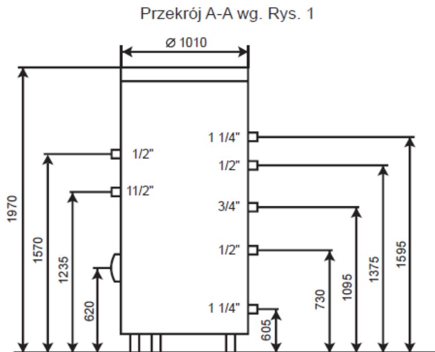
Rys.1 Budowa zasobnika SB750
