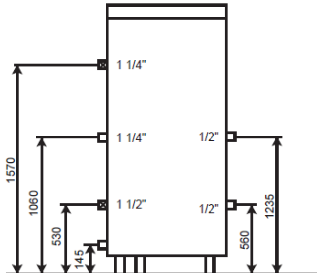
Rys. 2 Wymiary podgrzewacza
